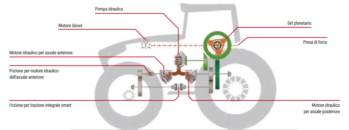
Lo schema della trasmissione del Fendt VarioDrive.
